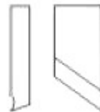
37° Beveling Tool
